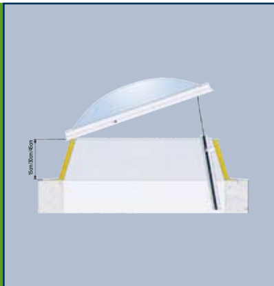
Wielkości świetlików kopułkowych ESSMANN typ 810
